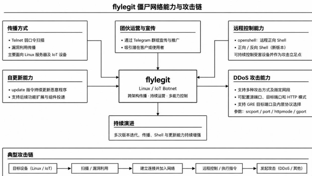
图 1 FlyLegit 僵尸网络能力与攻击链
